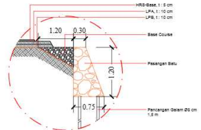
DETAIL POTONGAN Skala 1 : 50
