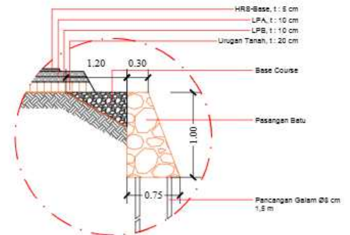
DETAIL POTONGAN Skala 1 : 50
