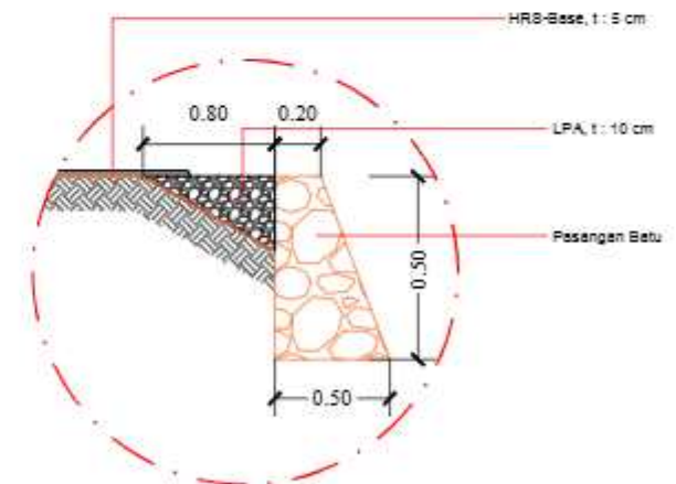
DETAIL POTONGAN Skala 1 : 50
